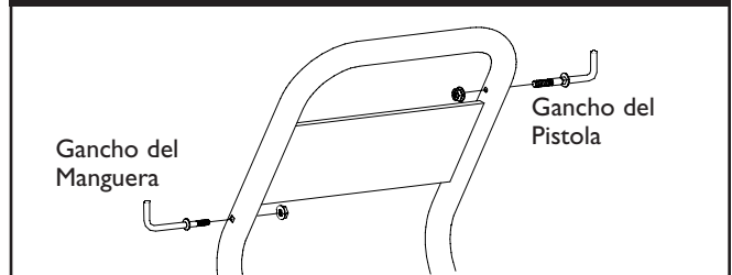
Figura 28 - Fijar el "L" Perno a la Manubrio
