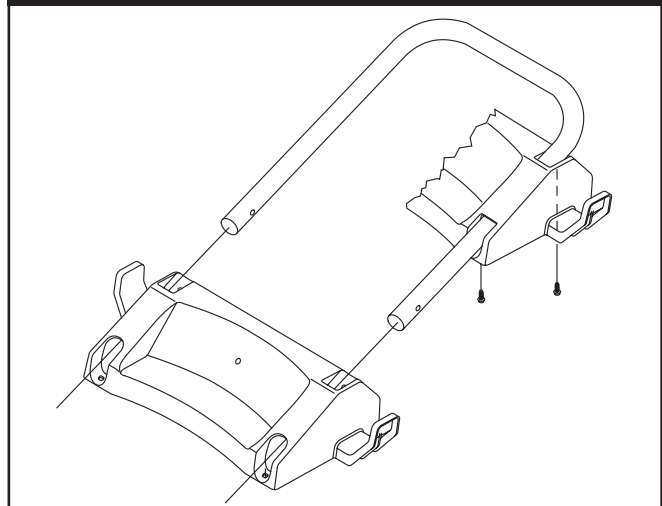
Figura 20 - Conecte Bandeja Accesorias
