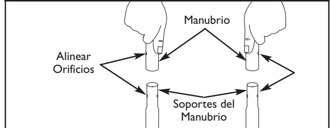
Figura 26 - Fijar el Manubrio a la Base
