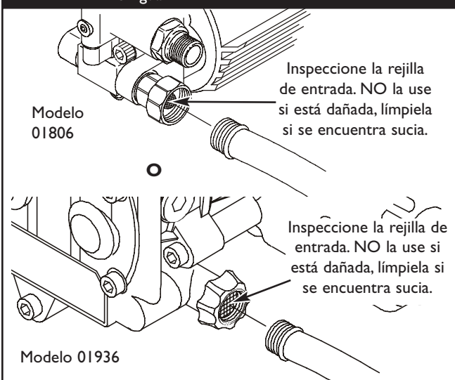
Figura 31 — Conecte la Manguera para el Jardín, a la Entrada de Agua
